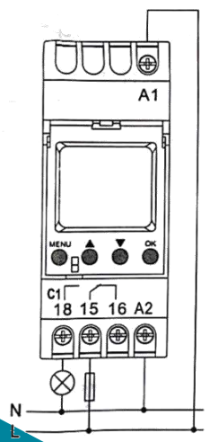
Conexión básico
