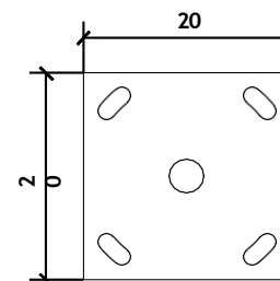
FLANCHE
