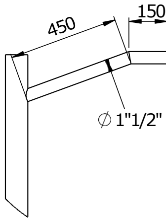
DETALLE a ESCALA 1 : 15
